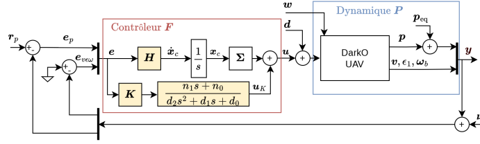
FIGURE 6.1 – Schéma de commande intégrale avec la perturbation de vent w , la perturbation du système à l'entrée d et à la sortie \nu .
