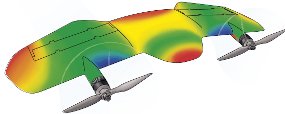
FIGURE 1.5 – Représentation de la pression dynamique sur la voilure de DarkO lors d'un vol d'avancement.
