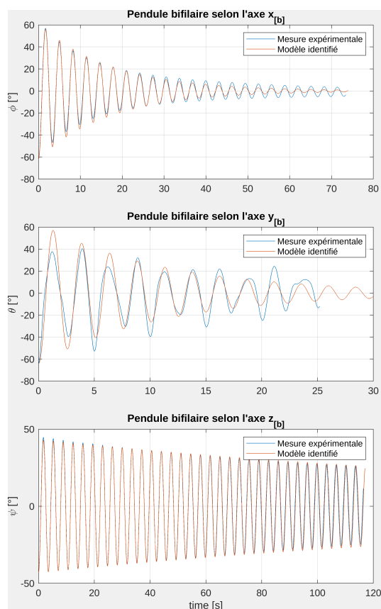
FIGURE 2.5 – Identification de l'inertie ( \mathbf{J} ), à partir des mesures issues du pendule bifilaire 2.4.
