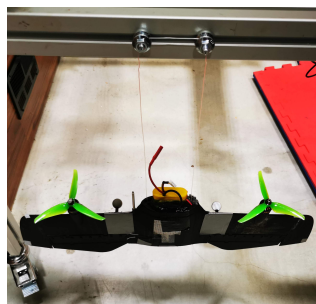
FIGURE 2.4 – Montage d'un pendule bifilaire pour l'identification de l'inertie ( \mathbf{J} ) de DarkO.
