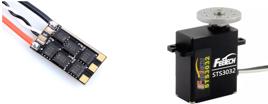
FIGURE 1.16 – Contrôleur moteur et servomoteur.
