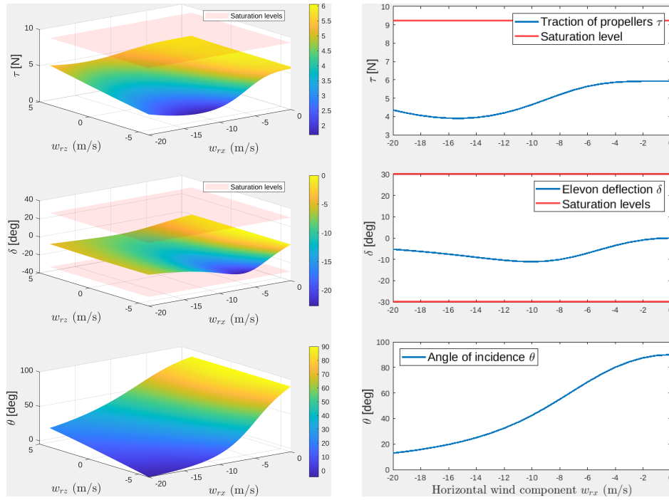
FIGURE 2.7 – Les paramètres (\tau, \delta, \theta) de l'ensemble des points d'équilibre (surface) obtenus à l'aide du Théorème 1 et de l'Algorithme 1 pour un vent constant horizontal et vertical (w_{rx}, w_{rz}) , avec les saturations des actionneurs (rose) (gauche) et coupe pour w_{rx} = 0 (droite).
