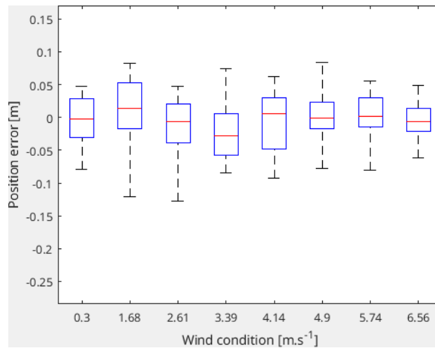
FIGURE 6.10 – Visualisation statistique des performances de vol stationnaire (en rouge la valeur moyenne, en bleu l'écart type à 95% et en pointillé les bornes minimales et maximales).
