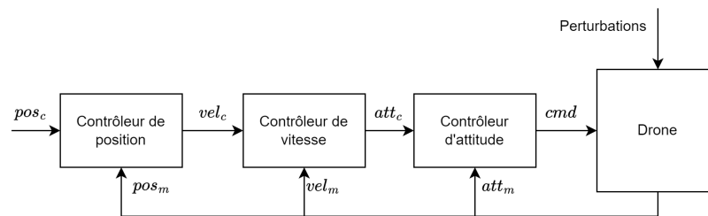
FIGURE 1.8 – Architecture classique de contrôle hiérarchique pour les drones.
