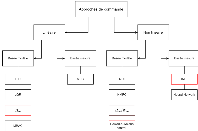
FIGURE 1.9 – Méthodes de commande utilisées sur les architectures tailsitter et freewing .
