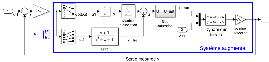
FIGURE 5.2 – Augmentation du système.
