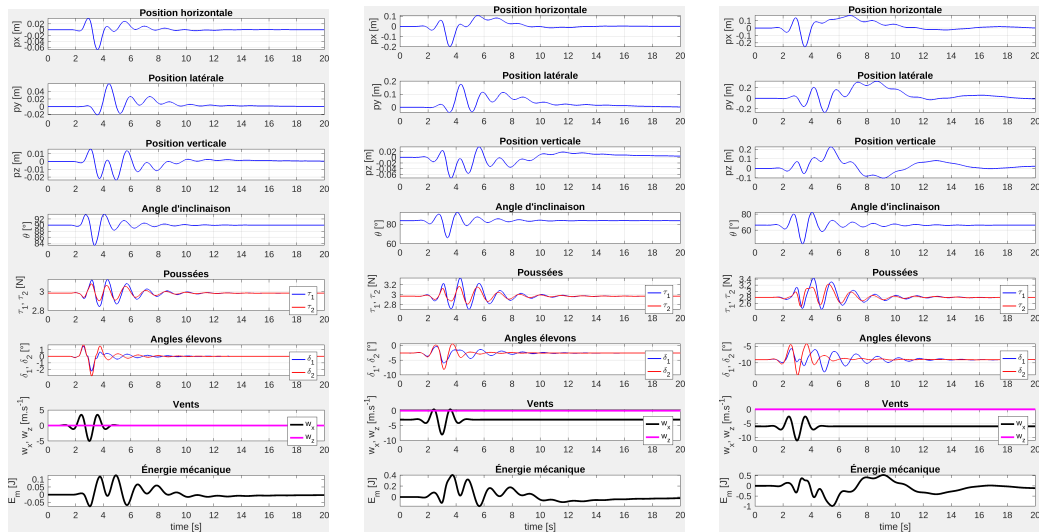
FIGURE 6.7 – Simulation du modèle non-linéaire (2.2) face à une perturbation "ondelettes de Morlet" (1.2).
