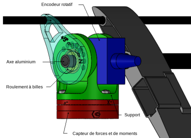
FIGURE 4.1 – Montage à un degré de liberté.
