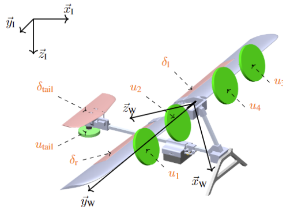
FIGURE 7.4 – Les repères, inertiel (I) et aile (W), attachés à l'architecture de Colibri.
