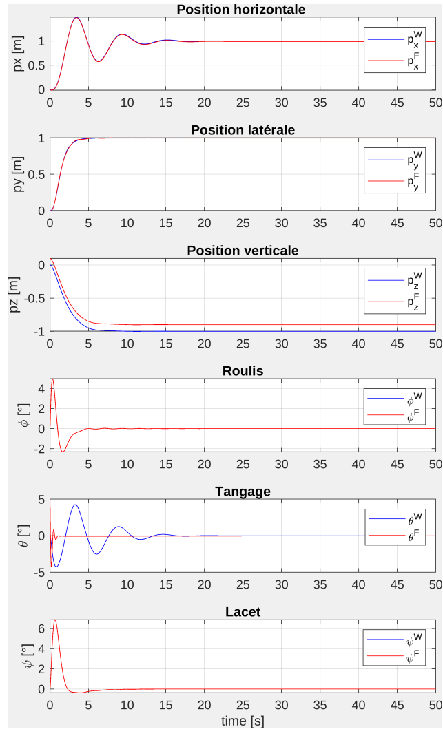
FIGURE 7.8 – Simulation de la position et de l'orientation du drone multicorps Colibri en boucle fermée avec un contrôleur à double boucle.
