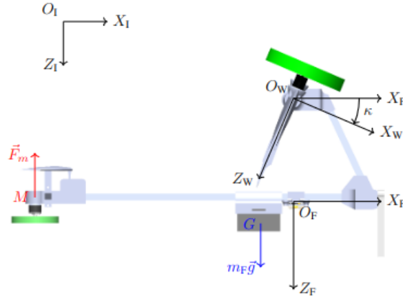
FIGURE 7.7 – Repère inertiel (I), du fuselage (F) et de l'aile (W) et forces agissant sur le drone Colibri.
