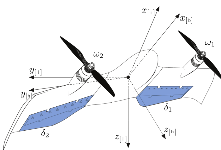
FIGURE 2.2 – Repère de référence de DarkO avec une représentation schématique des actionneurs.
