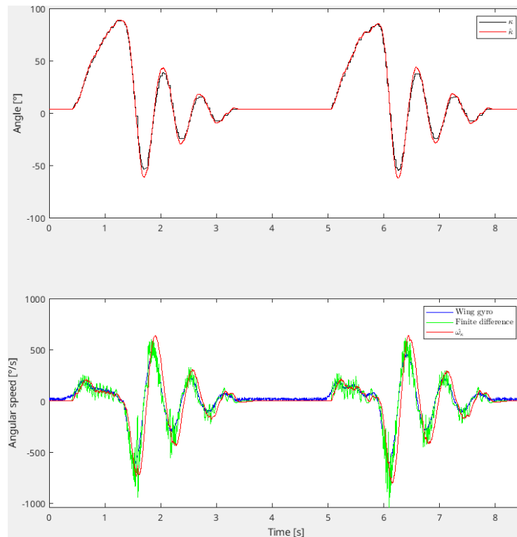
FIGURE 7.9 – Mesure de l'angle (noir, graphique du haut), mesure de la vitesse angulaire avec le gyroscope de l'aile (bleu, graphique du bas), estimation de la vitesse angulaire par différence finie (vert, graphique du bas) et estimation avec le filtre haut gain (courbes rouges).
