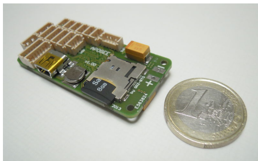
FIGURE 2.1 – Vue de dessus d'un autopilote Apogee v1.00.
