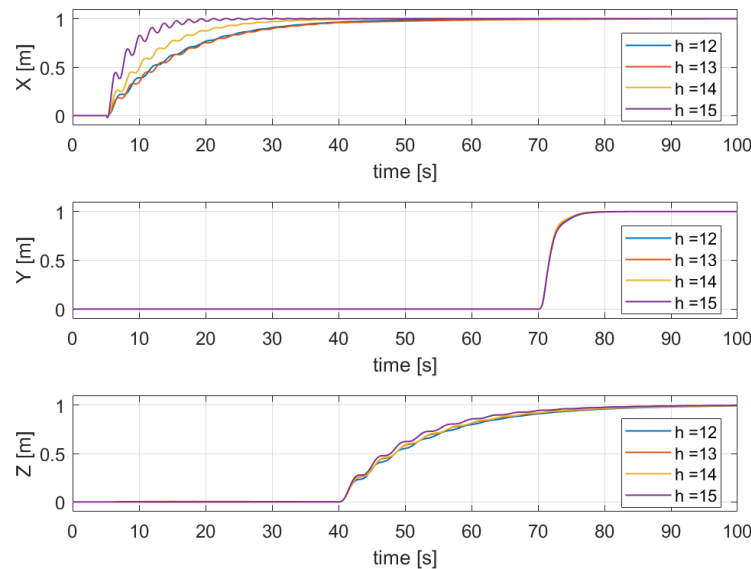
FIGURE 5.3 – Réponse du bouclage (5.13) avec une dynamique linéaire (2.30).
