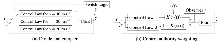
FIGURE 1.12 – Contrôleur séquencé discret (a) et continu (b) [Ducard 2021].
