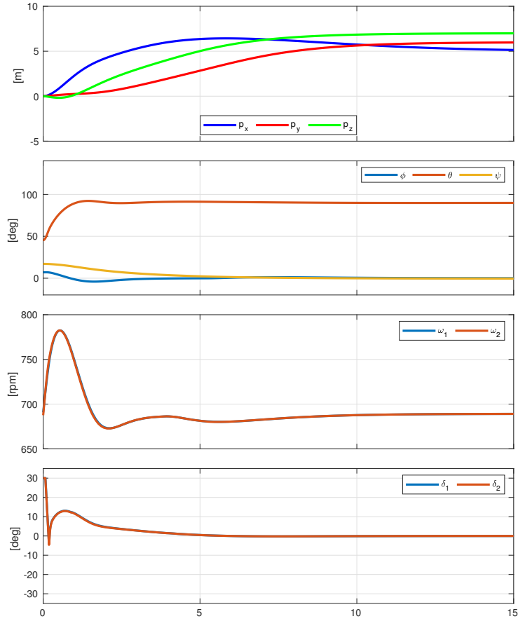
FIGURE 3.2 – Simulation de la loi de commande non-linéaire avec la dynamique de DarkO (2.2).
