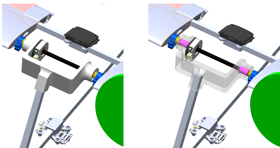
FIGURE 7.5 – Modèle 3D de la liaison.
