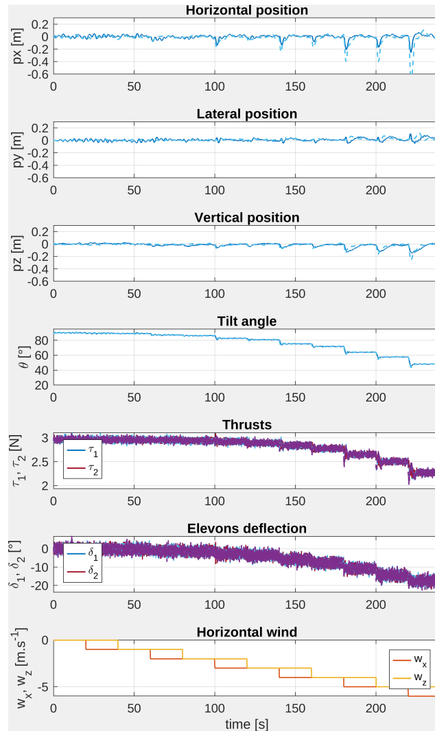
FIGURE 6.4 – Simulation du modèle non-linéaire (2.2) (ligne continue) et du modèle linéarisé (2.34) (ligne en pointillé) avec des incréments de vent constants croissants, le contrôleur étant réglé à l'aide de l'optimisation multimodèle de l'algorithme 3 dans la section 6.2.3.
