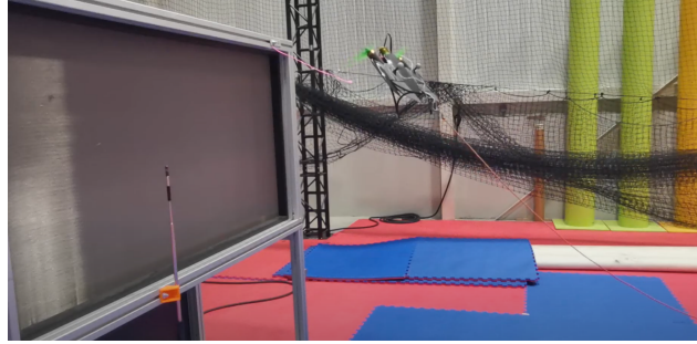
FIGURE 6.8 – Vol expérimental de DarkO devant la soufflerie ouverte.
