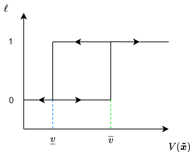
FIGURE 3.6 – Mécanisme d'hystérésis sur le changement local/global de loi de commande.
