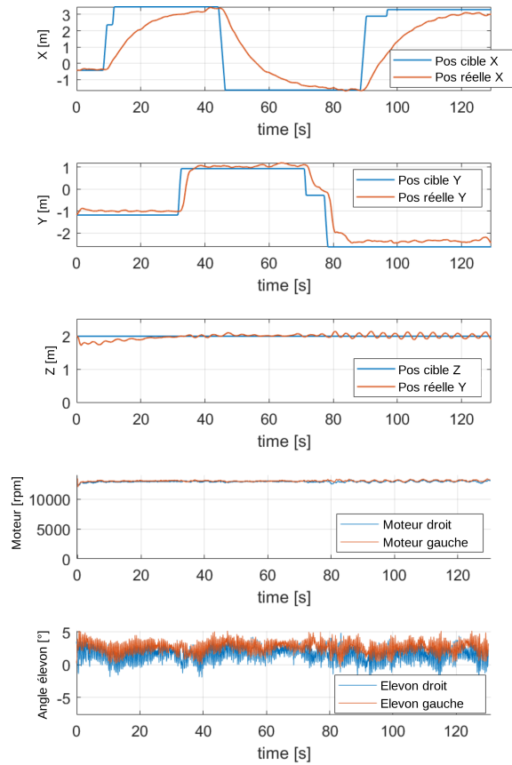
FIGURE 5.7 – Réponse expérimentale en boucle fermée et entrée de commande pour h = 12 .
