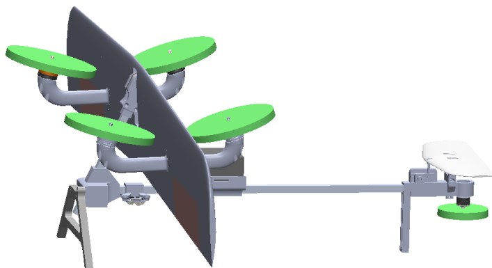
FIGURE 7.3 – Maquette de Colibri avec un montage des moteurs en H.
