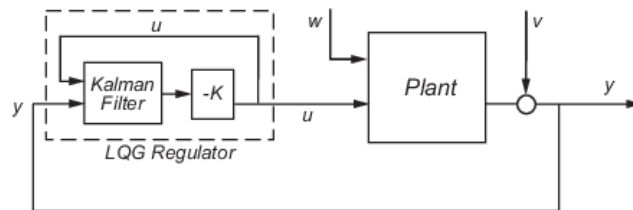
FIGURE 1.10 – Schéma de commande LQG.
