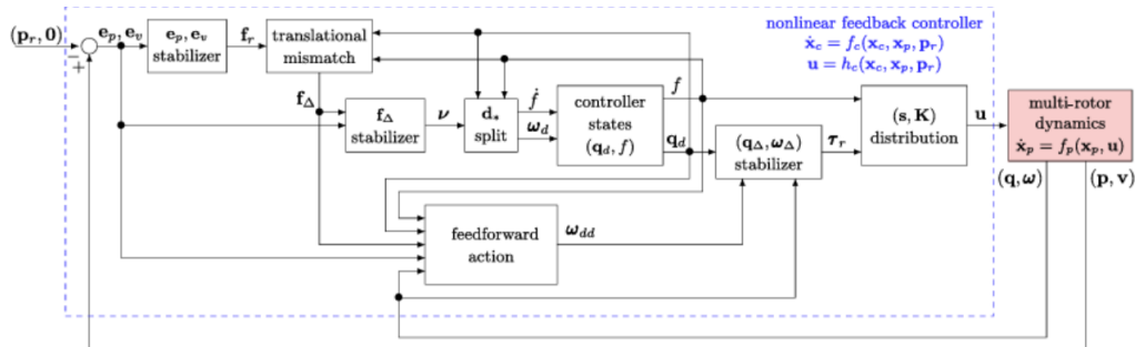
FIGURE 3.1 – Schéma de commande non-linéaire basée sur une direction de zéro moment [Michieletto 2020].
