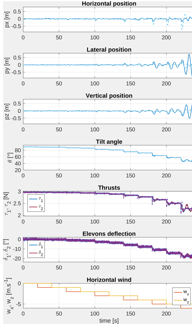
FIGURE 6.2 – Simulation du modèle non-linéaire (2.2) (ligne continue) et du modèle linéarisé (2.34) (ligne en pointillé) avec des incréments de vent constants croissants et le contrôleur basé sur l’optimisation sans vent de la section 6.2.2.
