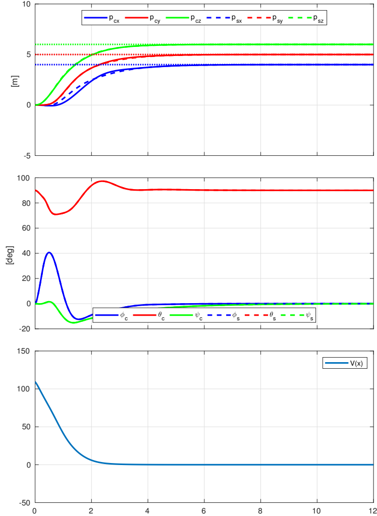
FIGURE 3.3 – Simulation du modèle complet (2.2) (ligne continue) et simplifié (2.15) (ligne en pointillé) avec \mathbf{u} = \mathbf{u}_{\text{lin}} défini dans (3.2) et comme condition initiale \tilde{\mathbf{x}}_0 dans le bassin d'attraction.
