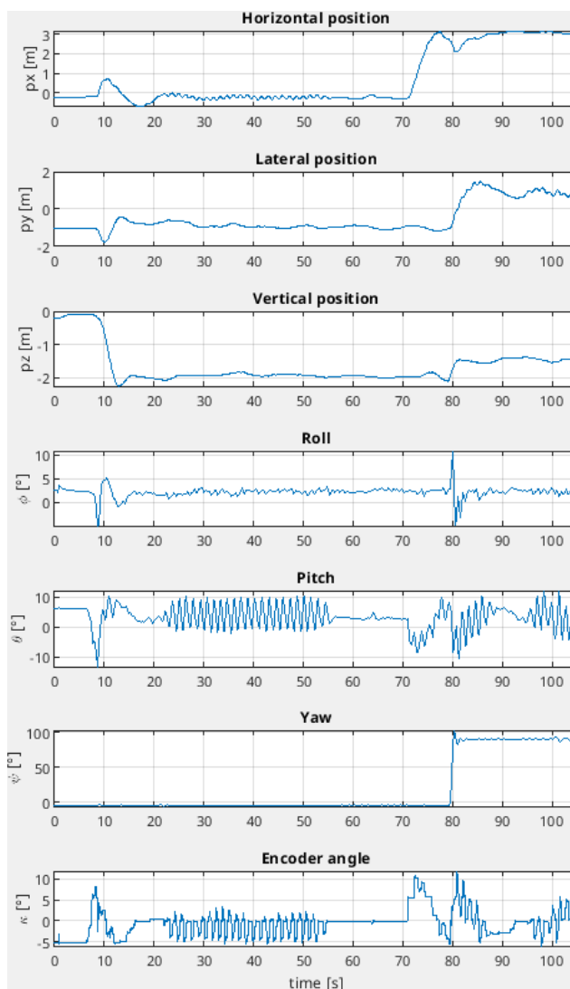
FIGURE 7.12 – Position et orientation de l’aile (six premiers graphiques) et mesure de l’angle entre l’aile et le fuselage (dernier graphique), lors d’un vol réel.
