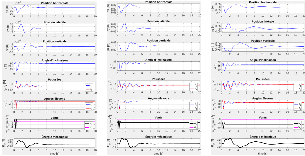
FIGURE 6.6 – Simulation du modèle non-linéaire (2.2) face à une perturbation "chapeau mexicain" (1.1) avec f_g = 1.2 Hz.
