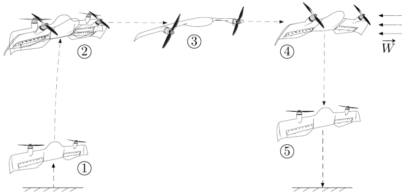
FIGURE I.1 – Phases de vol d'un drone tailsitter , DarkO.
