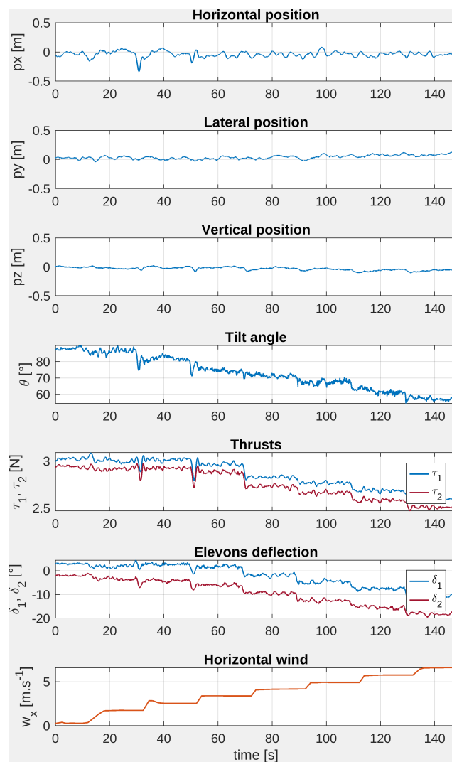
FIGURE 6.9 – Expérience du drone DarkO devant la soufflerie avec des incréments de vent constants croissants (graphique du bas).
