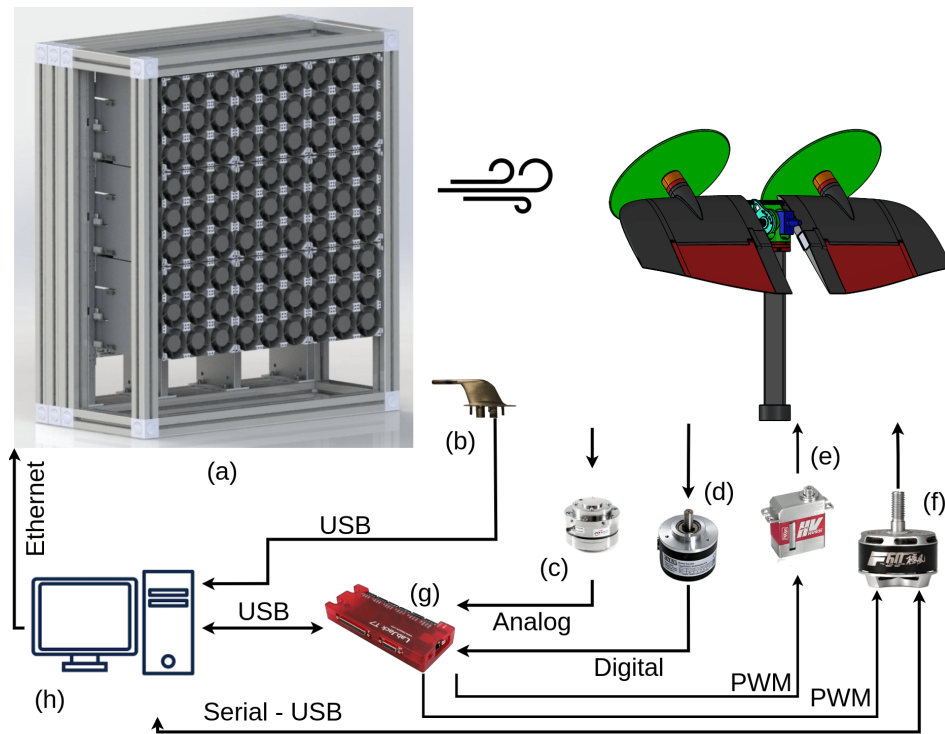
FIGURE 4.3 – Architecture d'essai en vol virtuel : WindShape (a) ; capteur de vitesse (b) ; capteur de forces et moments (c) ; encodeur rotatif (d) ; servomoteur (e) ; moteur brushless + ESC (f) ; LabJack (g) ; ordinateur de contrôle (h)
