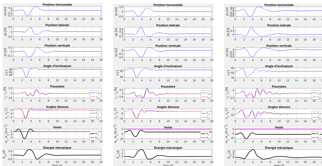
FIGURE 6.5 – Simulation du modèle non-linéaire (2.2) face à une perturbation "chapeau mexicain" (1.1) avec f_g = 0.2 \text{ Hz} .
