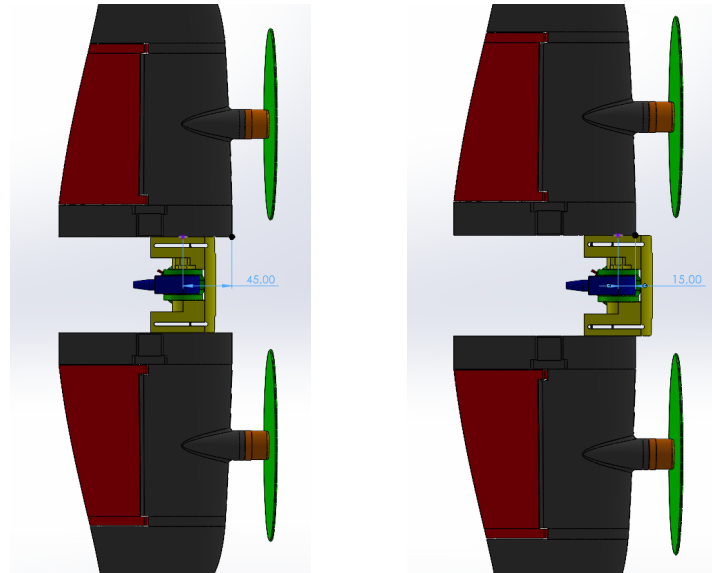
FIGURE 7.2 – Positionnement avant et arrière du centre de rotation par rapport au centre de gravité.
