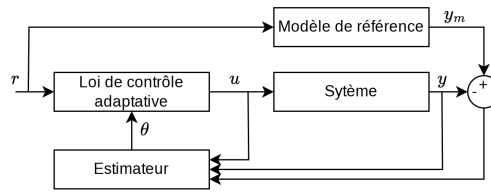
FIGURE 1.13 – Architecture d'un contrôleur MRAC.
