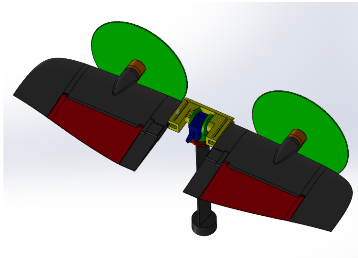
FIGURE 7.1 – Montage de la maquette du chapitre 4 avec un réglage de la position du centre de rotation (pièce jaune).
