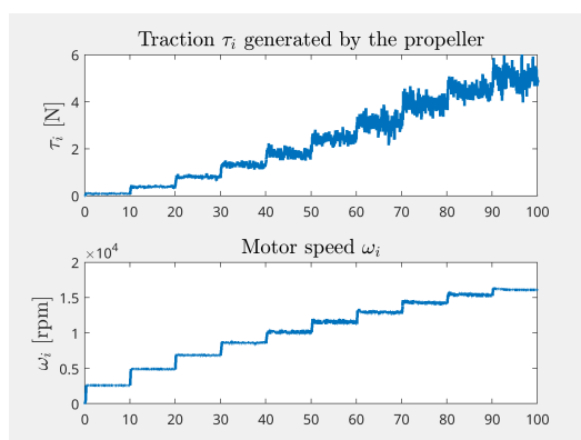
FIGURE 2.3 – Réponse entrée-sortie de l'ensemble moteur/hélice.
