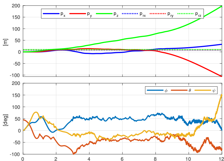
FIGURE 3.4 – Simulation divergente du modèle complet (2.2) avec \mathbf{u} = \mathbf{u}_{\text{lin}} défini dans (3.2) et une condition initiale \tilde{\mathbf{x}}_0 en dehors du bassin d'attraction.
