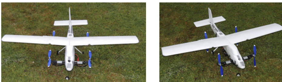
FIGURE 1.2 – Structure Tiltrotor proposée par [Flores 2014], dans deux configurations, vol stationnaire et d'avancement.
