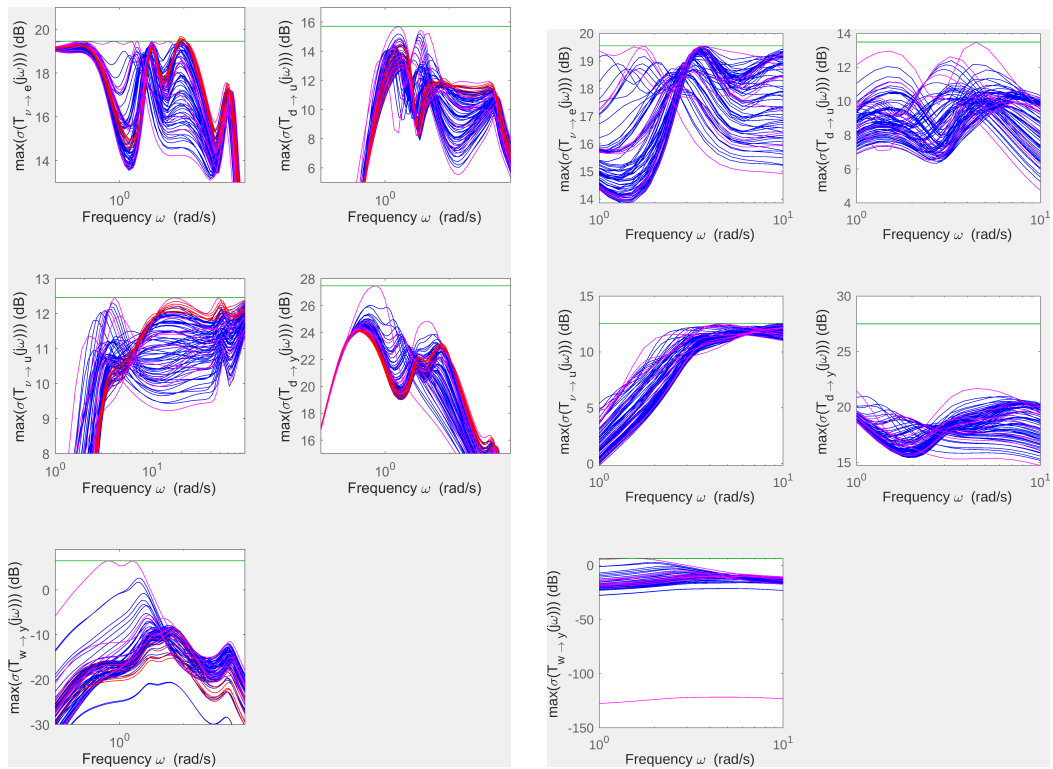
FIGURE 6.3 – Diagrammes des valeurs singulières des fonctions de transfert dans (6.8), à la première itération de l'algorithme 3 (à gauche) et à la seconde itération (à droite).
