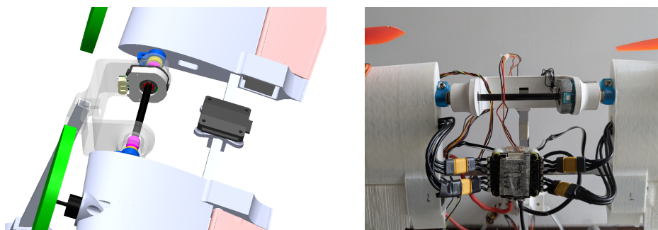
FIGURE 7.6 – Visualisation de l'encodeur rotatif sur le modèle 3D (gauche) et modèle réel (droite).
