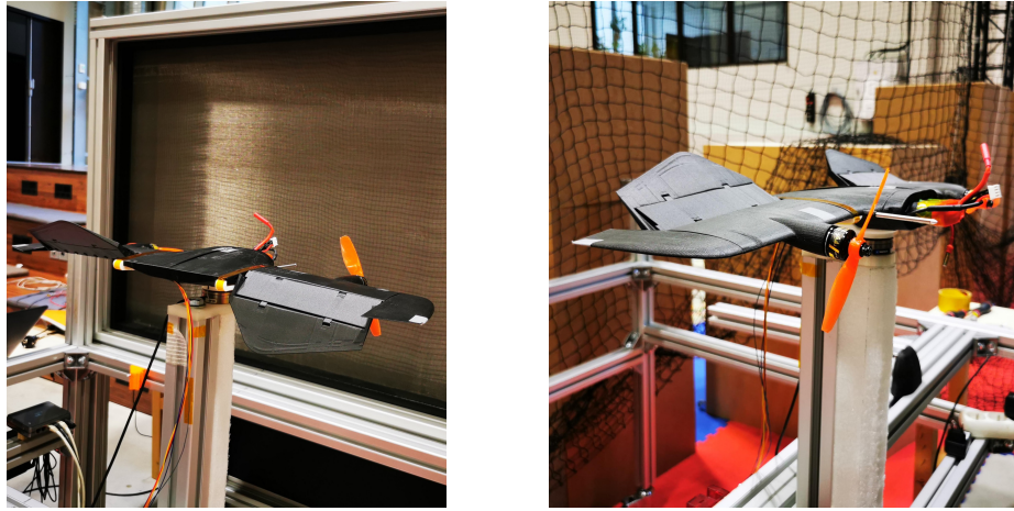
FIGURE 2.6 – Montage de DarkO sur un banc de mesure face à une soufflerie ouverte.
