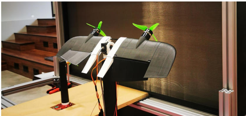
FIGURE 4.2 – Modèle de DarkO à un seul degré de liberté devant le WindShape .
