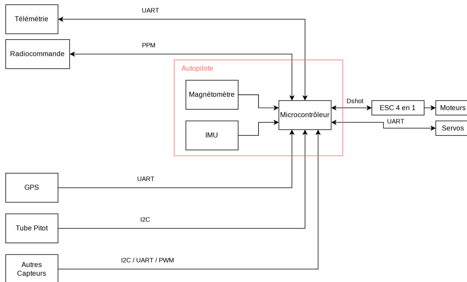
FIGURE 1.15 – Architecture d'un autopilote et son environnement.
