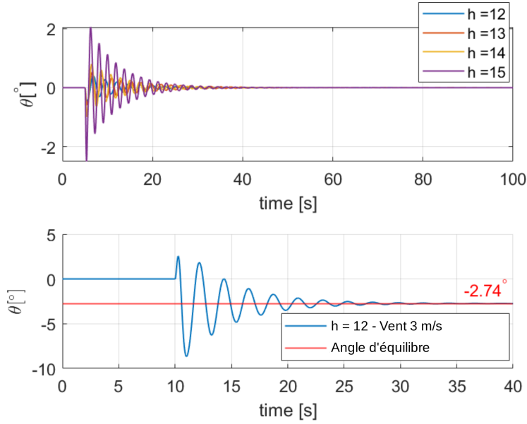
FIGURE 5.4 – Réponse temporelle de l'angle d'incidence \theta en boucle fermée.
