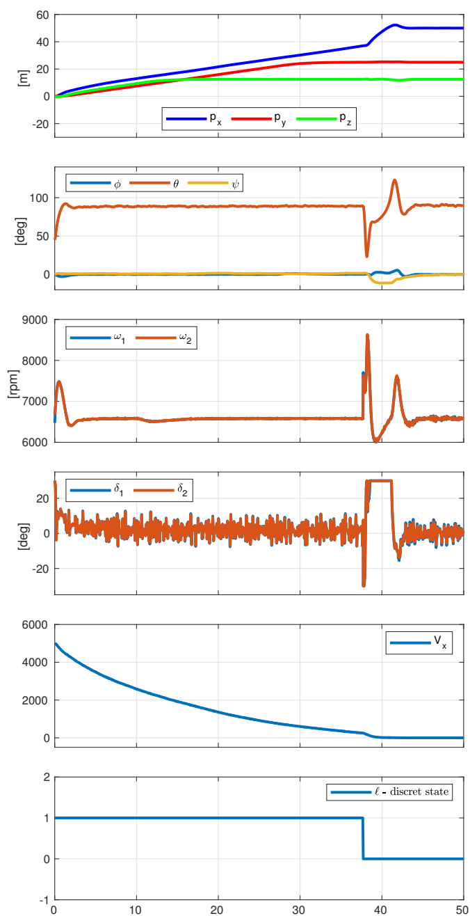
FIGURE 3.7 – Simulation en boucle fermée avec le contrôleur hybride (3.4).
