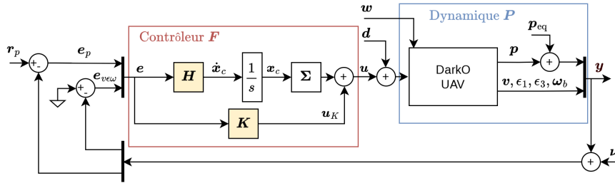
FIGURE 4.4 – Schéma de commande linéaire, proportionnelle-intégrale.
