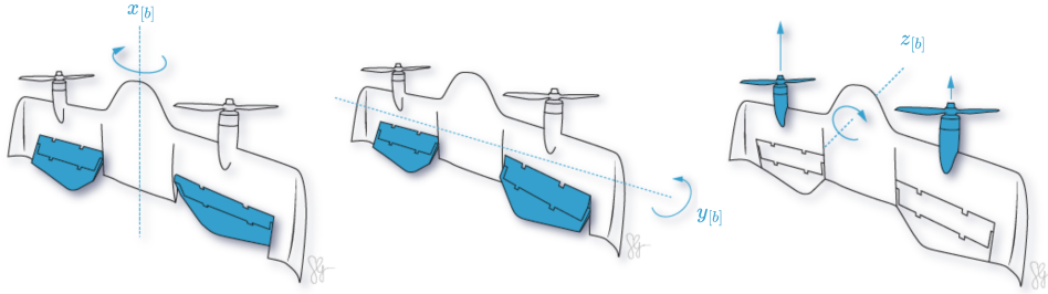
FIGURE 1.7 – Actionneurs d'un tailsitter et leurs actions sur les axes principaux.
