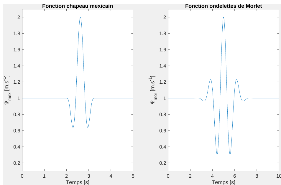
FIGURE 1.6 – Représentation temporelle des modèles de perturbation de vent.
