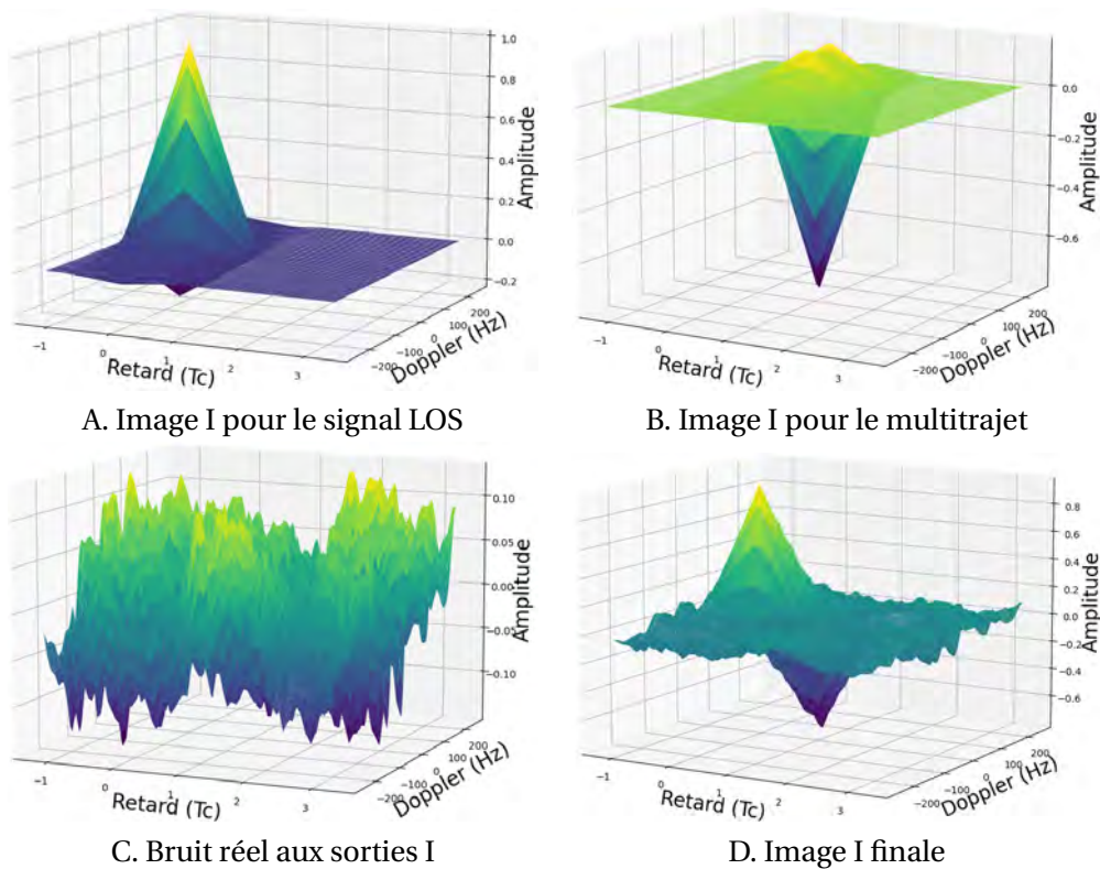
FIGURE 2.9 – Génération des différentes sorties de corrélateur pour la composante I d’un signal subissant un multitrajet de paramètres \tau_{MP} = 0.75 T_c , \delta f = 50 Hz, \alpha_{MP} = 0.8 et \phi_{MP} = \pi .
