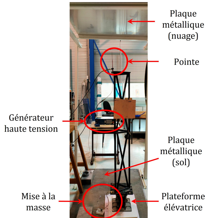
FIGURE 4.1 – Photo du montage expérimental
