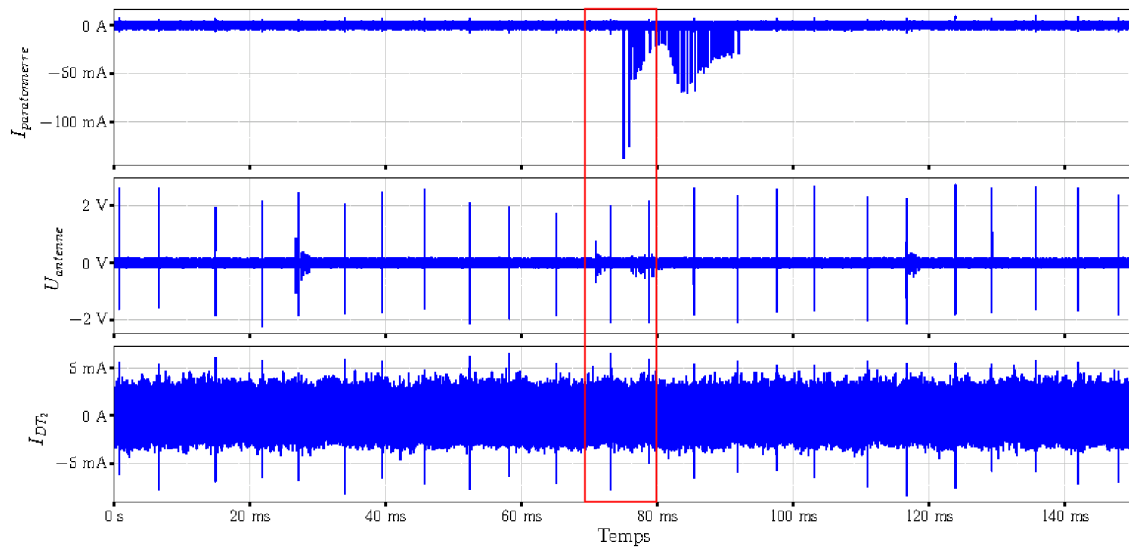
FIGURE 3.35 – Enregistrement d'une acquisition du 24 juin 2022 à 7h05 avec le Picoscope 5244D
