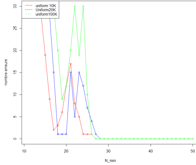
FIGURE 5.1 – Évolution en fonction de N_{\min} (décroissant) du nombre d'échecs de clustering (sur 30 essais) pour trois échantillons répartis selon la même loi uniforme mais dont le nombre d'observations est 10 000, 20 000 et 100 000.
