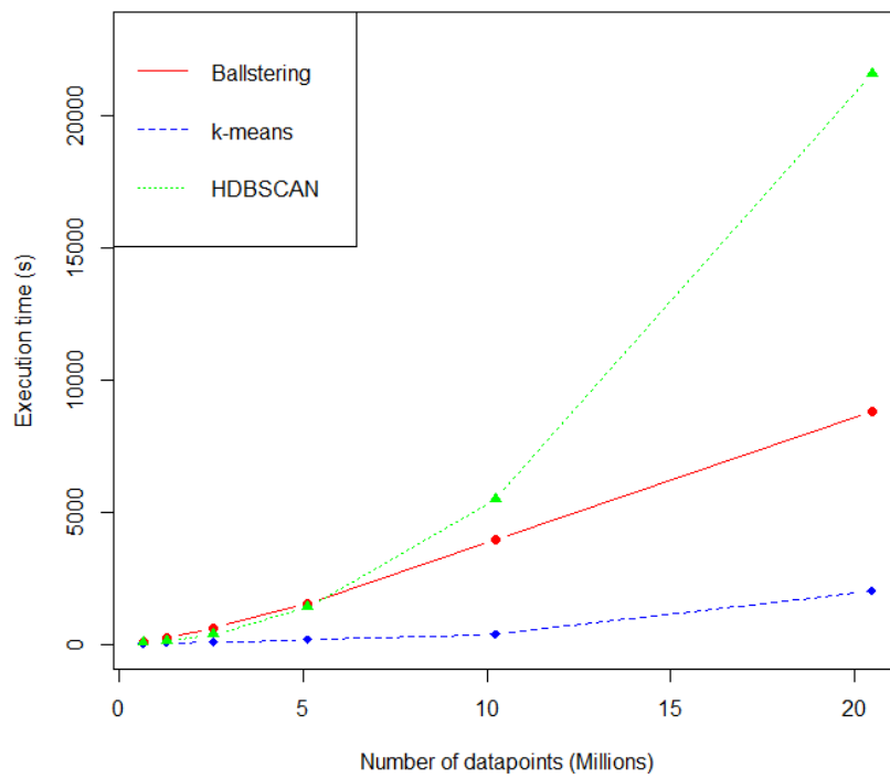
FIGURE 6.5 – Temps d'exécution de Ballstering, HDBSCAN et k -means lorsque le nombre d'observation augmente.
