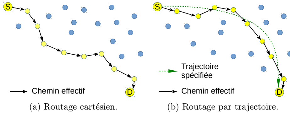
FIGURE 3.5 – Illustration du fonctionnement d’algorithmes de routage géographique.
