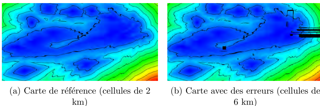
FIGURE B.1 – Cartes des temps de propagation
