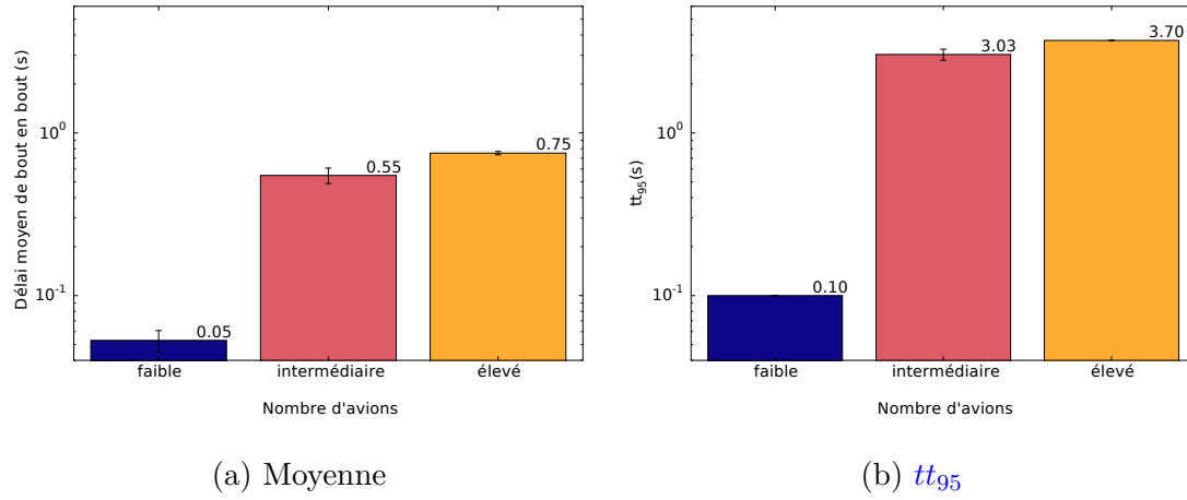
FIGURE 4.8 – Délai de bout en bout.
