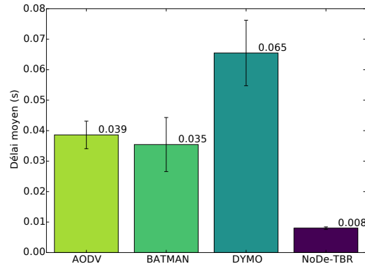
(b) Délai de bout en bout
