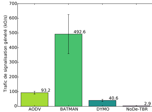
(a) Volume du trafic de signalisation généré
