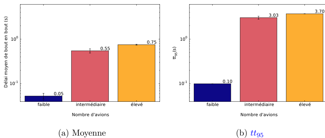
FIGURE 4.8 – Délai de bout en bout.
