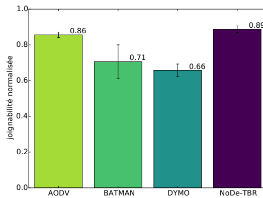
(c) Joignabilité normalisée
