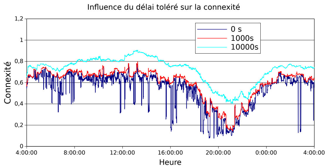
FIGURE 3.4 – Connectivité au cours de la journée en fonction de la durée de déconnexion tolérée (zone océanique, portée de 200 km).
