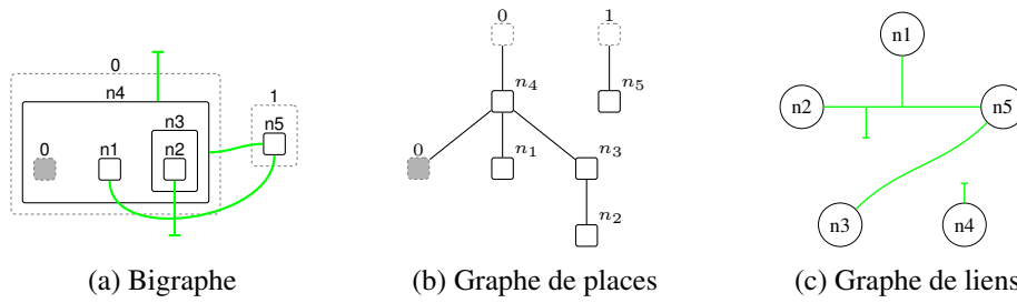
FIGURE 1 – Un bigraphe et sa décomposition en graphes de places et de liens
