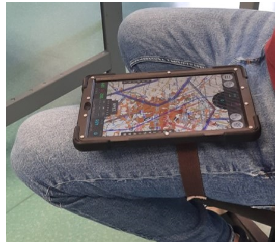
FIGURE 9: Tablette fixée par un kneebord
