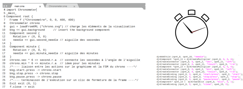
Figure 1: Code Smala, extrait du code C/Djnn et résultat de l'exécution d'un chronomètre
