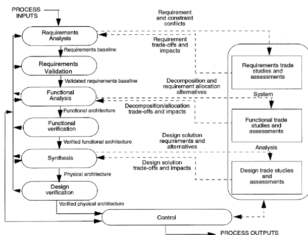
Figure 2: les processus d'ingénierie système selon la norme IEEE 1220-2005
