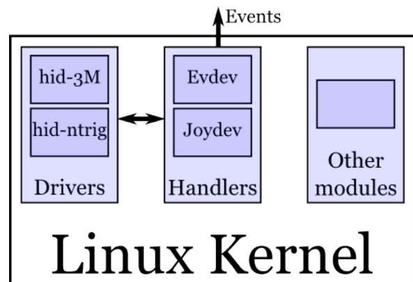
Figure 1. Gestion des entres multi-tactiles dans le noyau Linux
