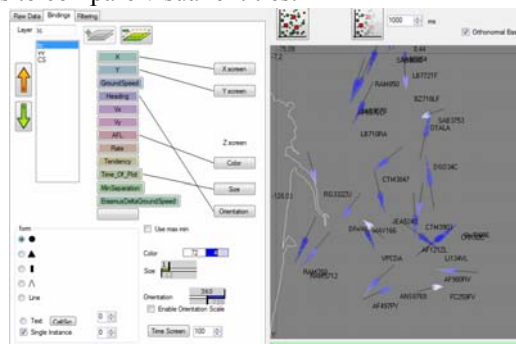
Fig. 5 : dataflow implementation
