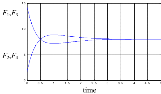
Fig. 3 Hover control inputs
